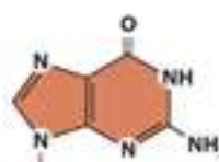
Guanin G
