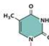
Tymin T
